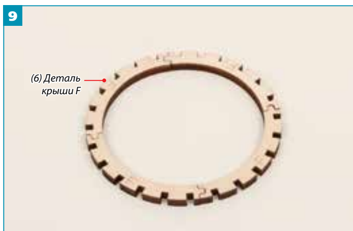
9 Присоедините оставшуюся маленькую деталь крыши F. Таким образом мы получили верхнюю часть каркаса крыши.
